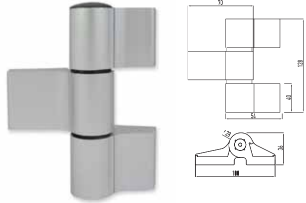
AL-073-B Colours / Boya Özellikleri Technical Information / Teknik Bilgi C-60 Hinge Oval Style Ral, Eloksal C-60 3"lü Menteşe
