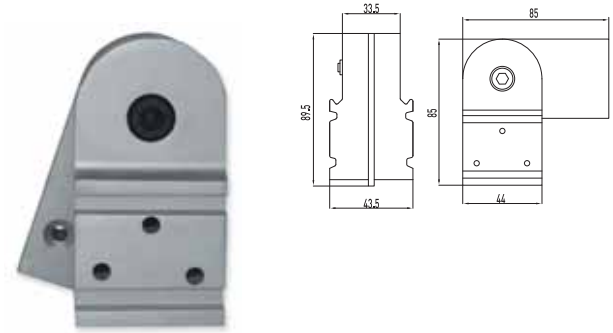
AL-076-A Colours / Boya Özellikleri Technical Information / Teknik Bilgi Spin Hinge Ral, Eloksal Pivot Menteşe Nal Model
