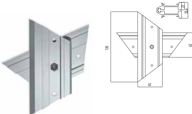
AL-076-C Colours / Boya Özellikleri Technical Information / Teknik Bilgi Spin Hinge Heat Insulated Ral, Eloksal Pivot Menteşe Üçgen Isı Yalıtım
