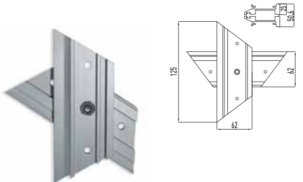
AL-076-B Colours / Boya Özellikleri Technical Information / Teknik Bilgi Spin Hinge Aldox Ral, Eloksal Pivot Menteşe Üçgen Aldoks
