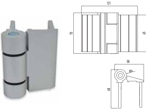
AL-071-C Colours / Boya Özellikleri Technical Information / Teknik Bilgi C-60 Fitted Hinge Ral, Eloksal C-60 Baba Menteşe
